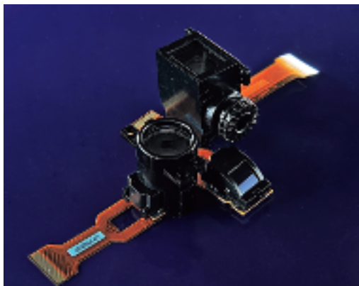
▲デジタルカメラ用電子ビューファインダー
