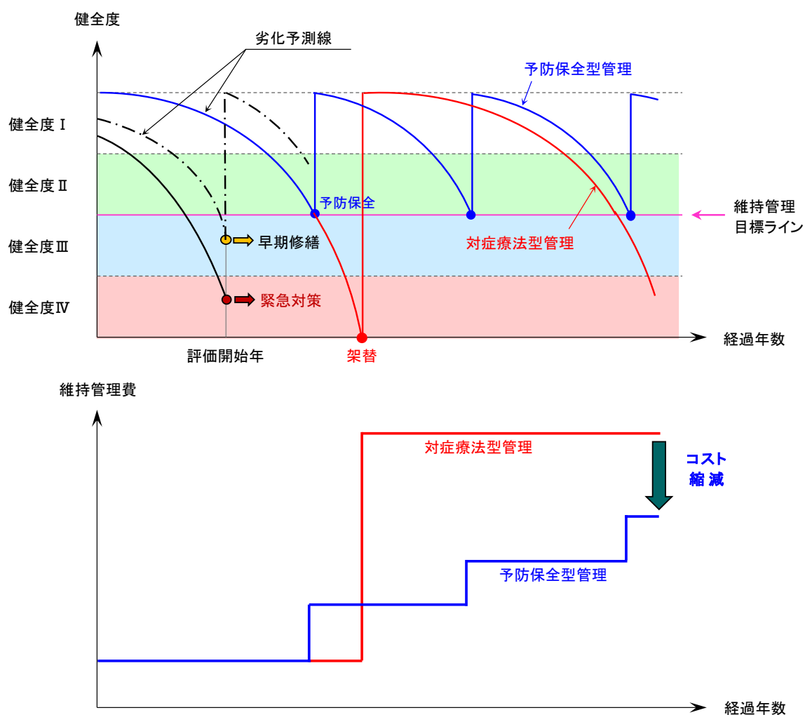
【管理手法による健全度と維持管理費の変移イメージ図】
