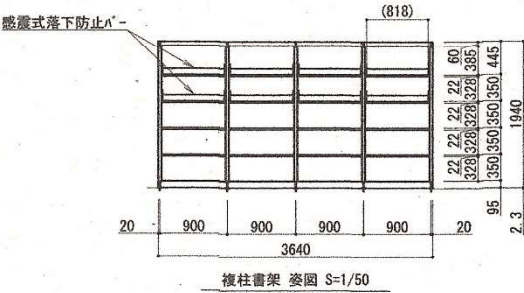
複柱書架 姿図 S=1/50
