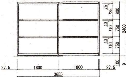
中量ホトリスラック 姿図 S=1/50
