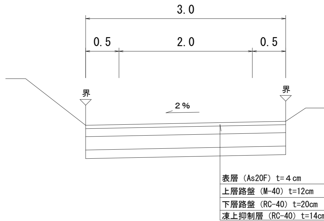
標準横断図 (S=1/50)
