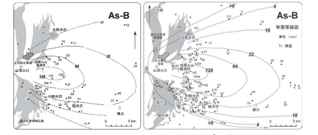
2015年以前 2016年プロジェクト開始後(2018年12月時点) 天仁噴火の火山灰分布図の違い 提供：安井真也
